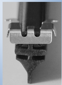
Abb. 1 Standard-Gummi mit Metallklammer
